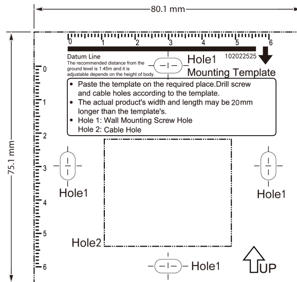
Рисунок 3-2. Монтажный шаблон
