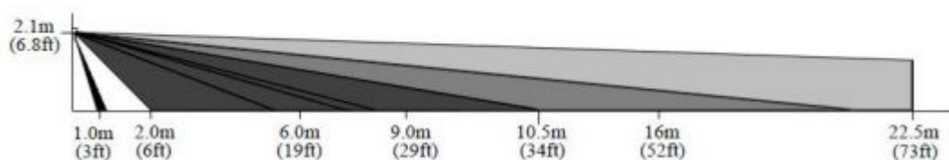
Рис. 5 Диаграмма зоны обнаружения АОПИ-Штора
