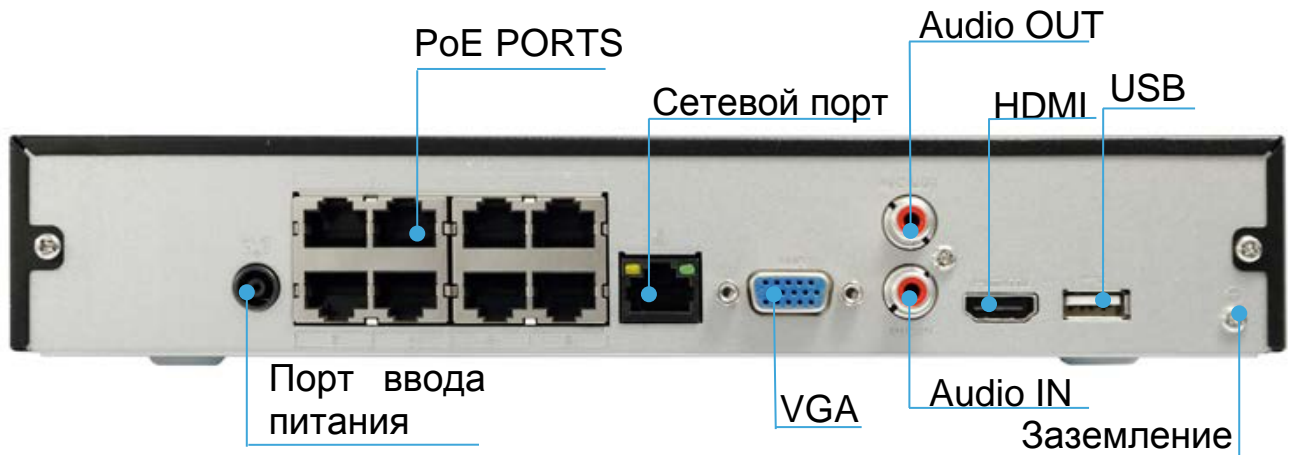
Рисунок 3.2 – Внешний вид задней панели
