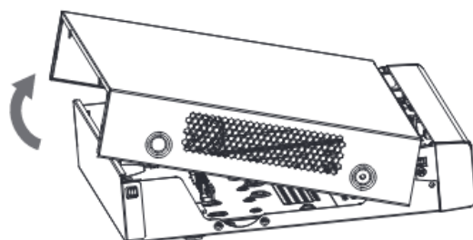
Рисунок 3.4 – Установка жесткого диска
