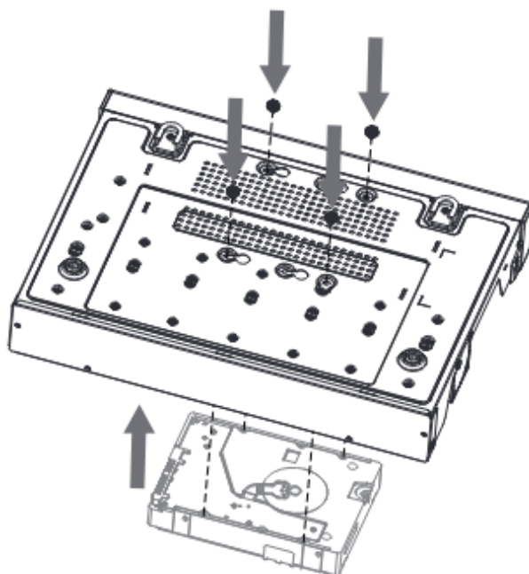
Рисунок 3.5 – Установка жесткого диска
