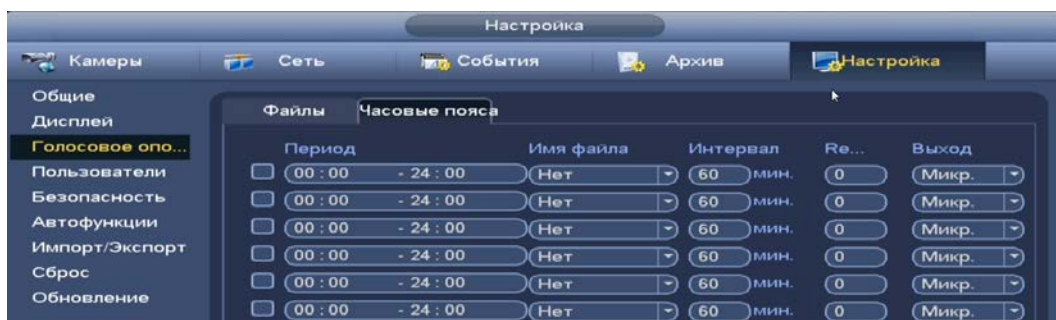
Рисунок 8.1 – Расписание
