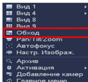
Рисунок 6.3 – Контекстное меню
