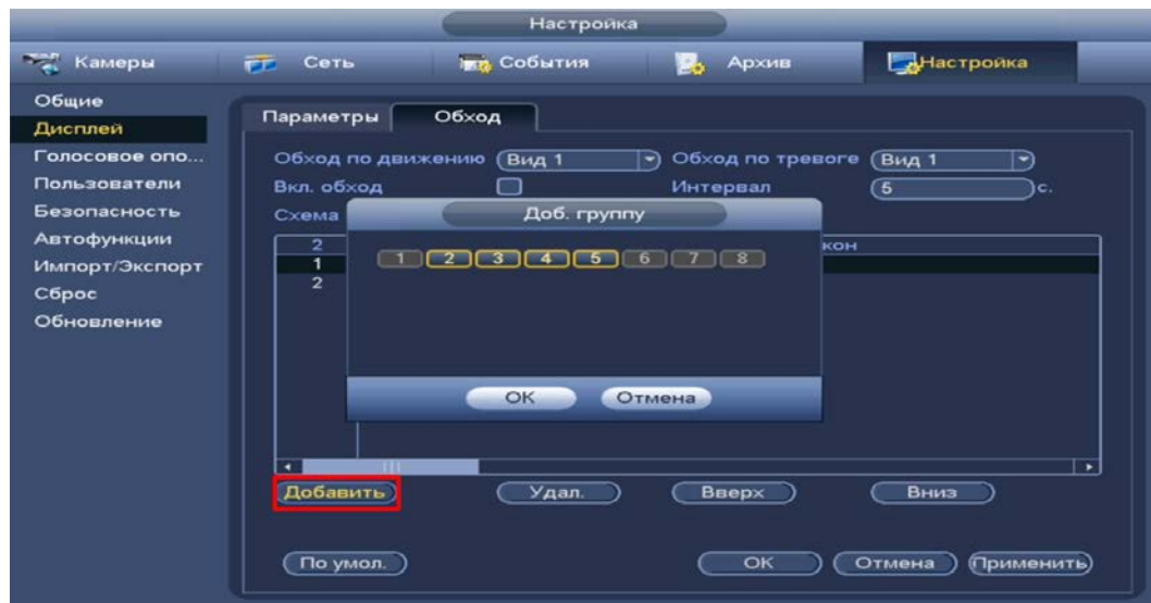
Рисунок 7.7 – Добавление группы
