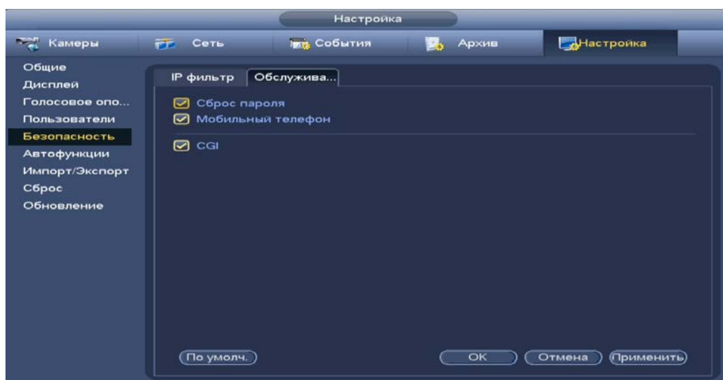
Рисунок 16.13 – Системное обслуживание
