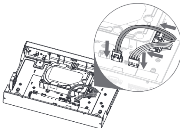
Рисунок 3.6 – Установка жесткого диска
