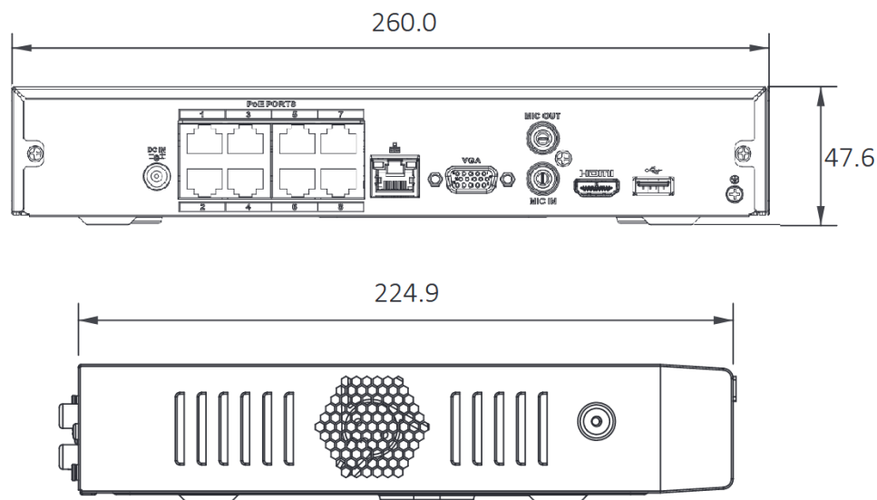
Рисунок 3.8 – Габаритные размеры видеорегистратора
