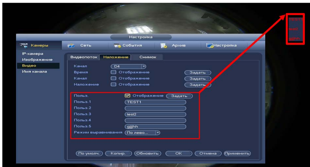
Рисунок 12.6 – Текстовое наложение
