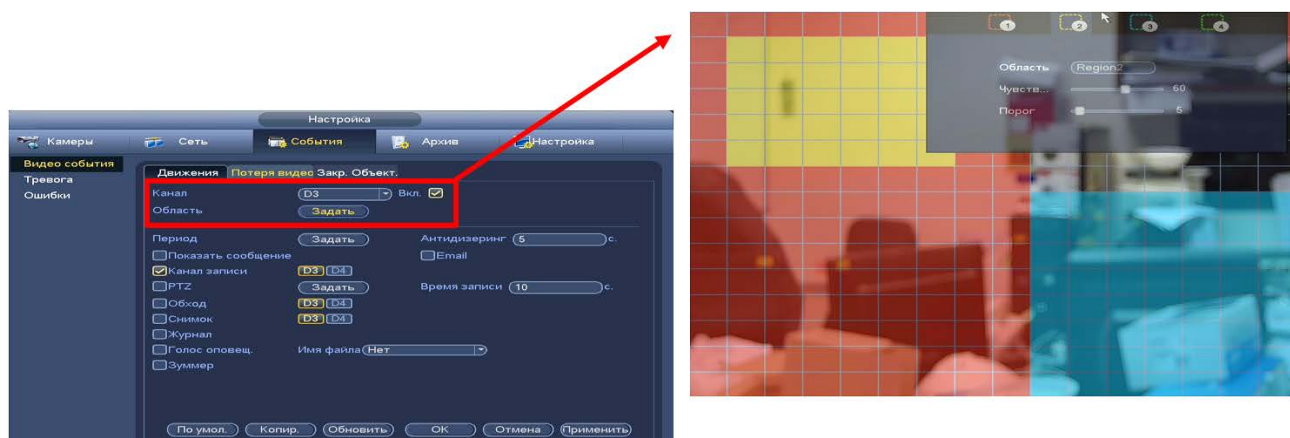
Рисунок 13.1 – Настройка области
