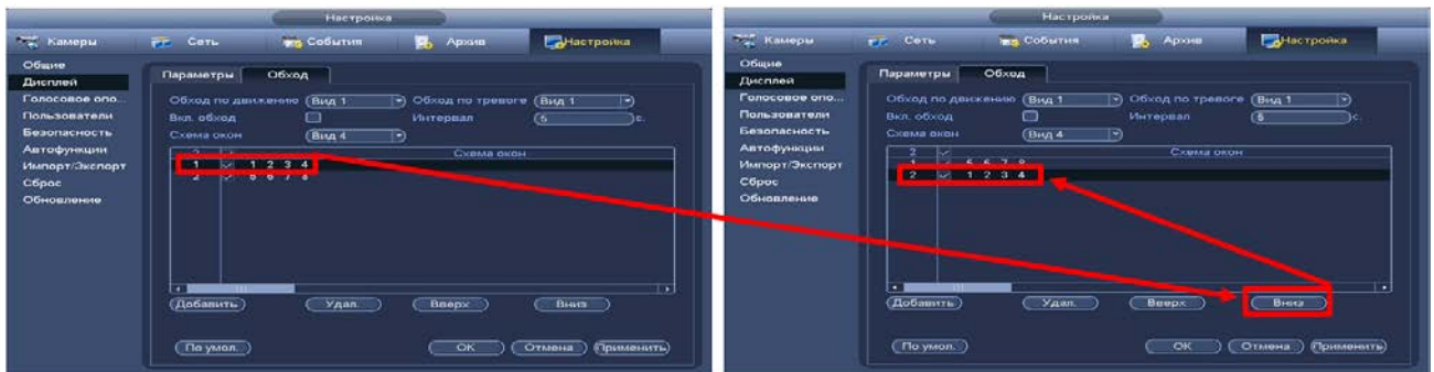
Рисунок 7.6 – Расположение групп
