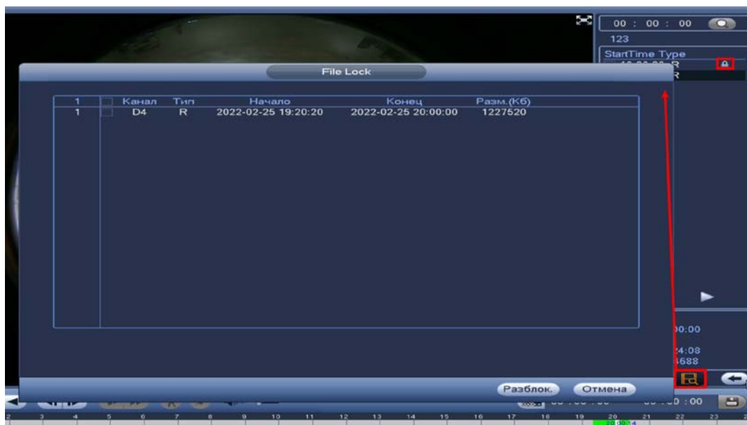
Рисунок 15.10 – Блокировка/Разблокировка файлов
