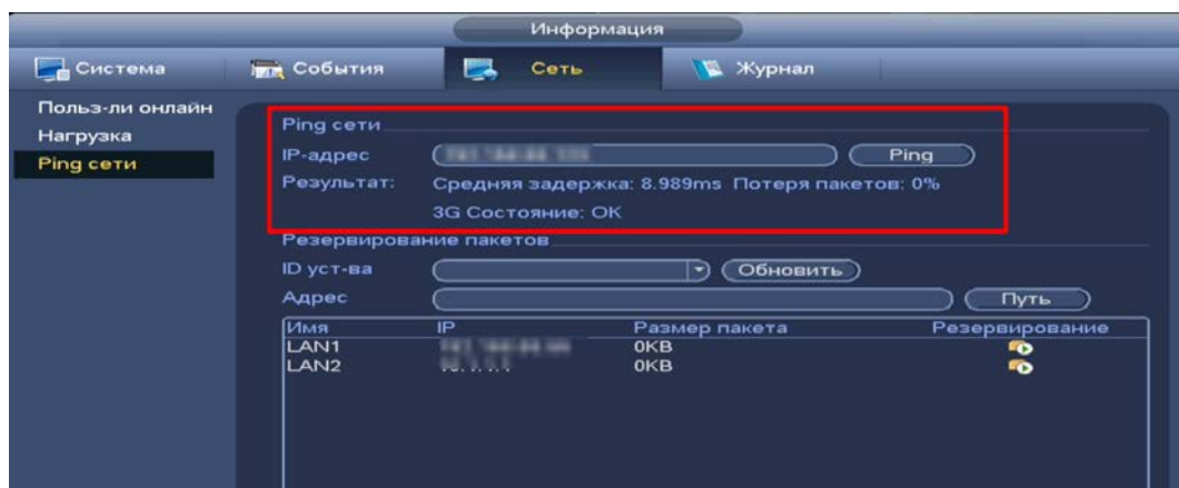
Рисунок 10.16 – Проверка IP-адреса
