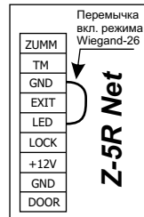
Рис.4 Установка переключателя для представления ключей в формате Wiegand-26
