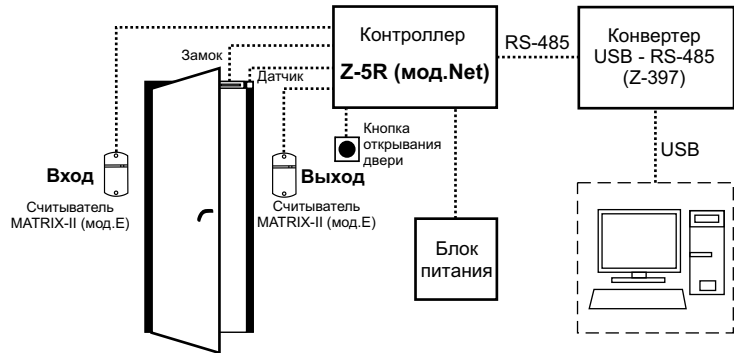
Рис.1 Схема СКУД с контроллером Z-5R (мод.Net)
