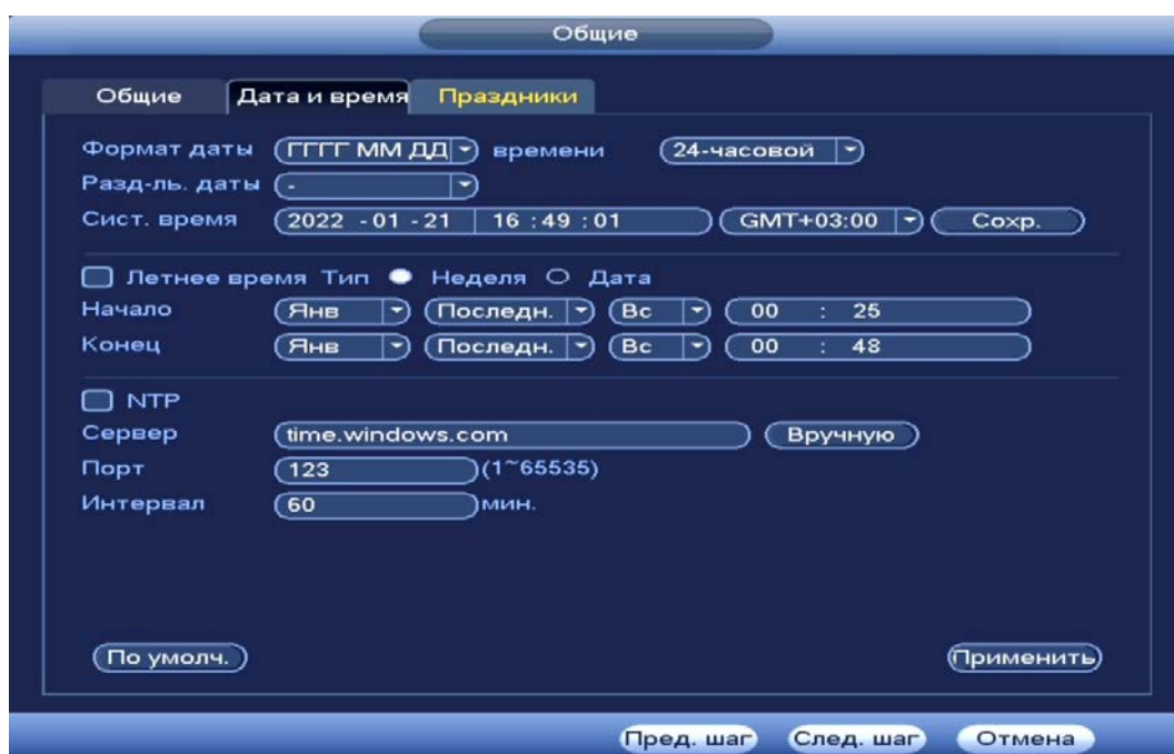
Рисунок 5.2 – Интерфейс меню быстрой настройки «Дата и время»
