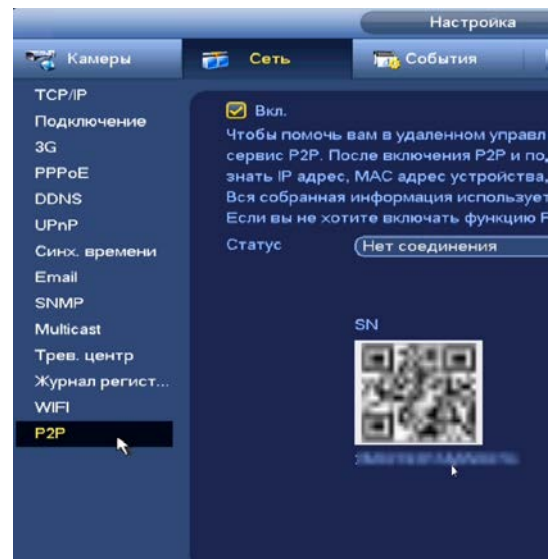
Рисунок 10.19 – QR-код добавляемого устройства
