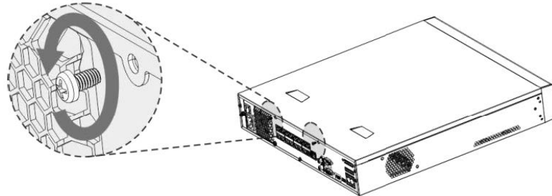
Рисунок 3.3 – Установка жесткого диска
