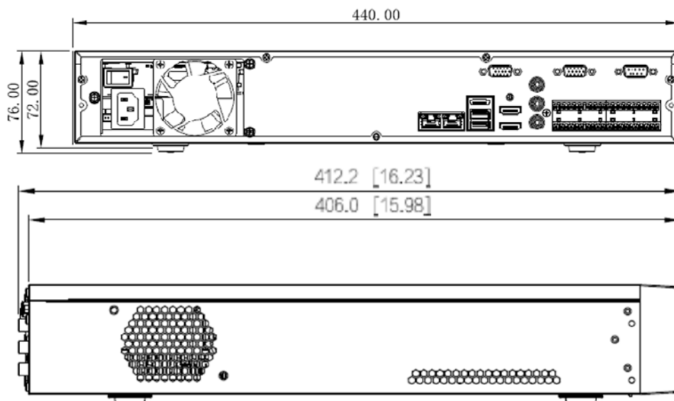
Рисунок 3.10 – Габаритные размеры видеорегистратора
