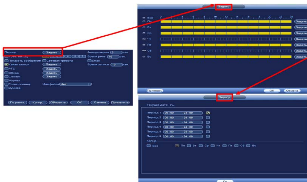
Рисунок 18.26 – Расписание
