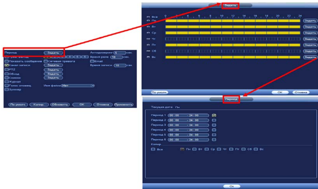
Рисунок 18.29 – Расписание
