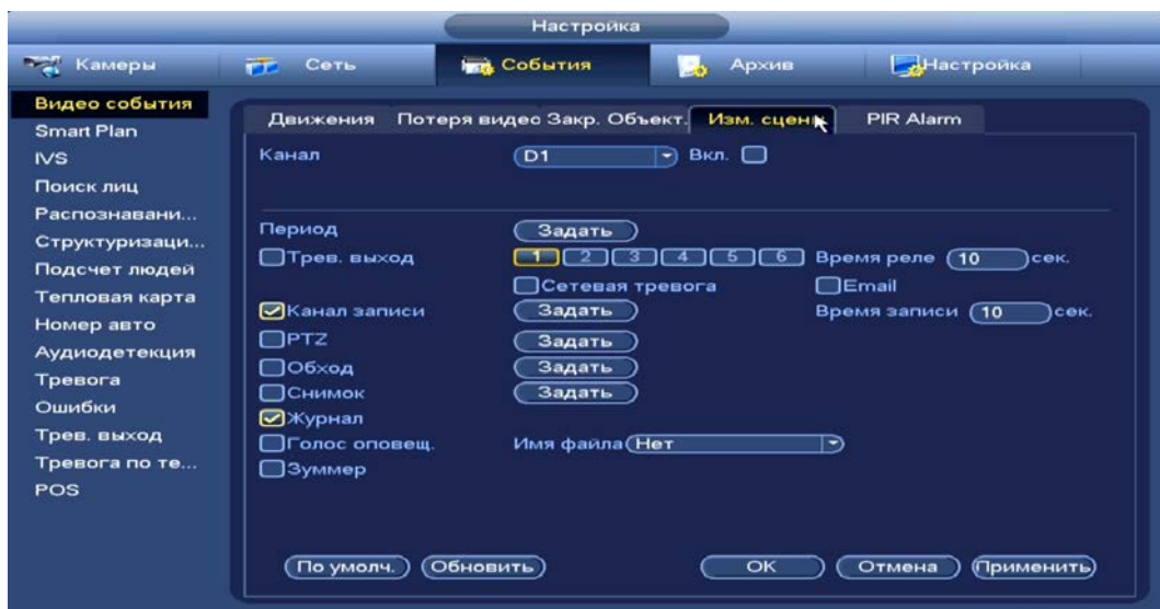
Рисунок 14.8 – Настройка события
