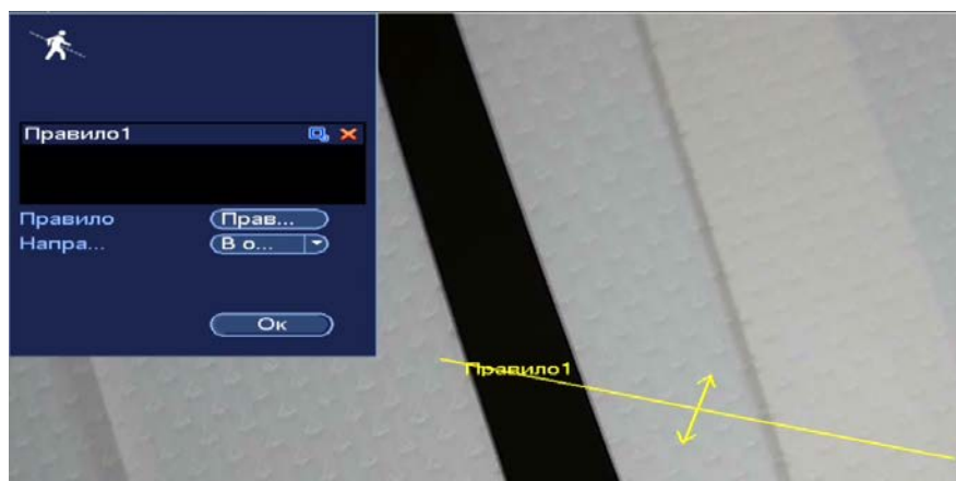
Рисунок 18.3 – Настройка правила
