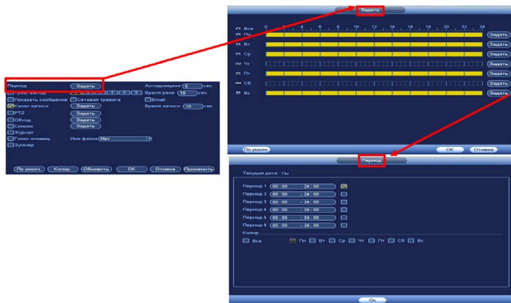
Рисунок 14.15 – Расписание
