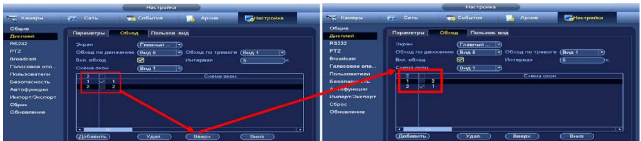
Рисунок 8.6 – Расположение групп
