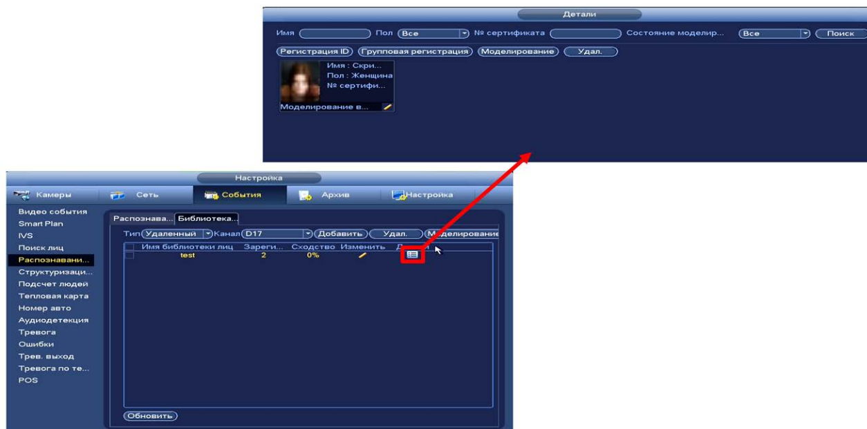
Рисунок 18.18 – Библиотека лиц
