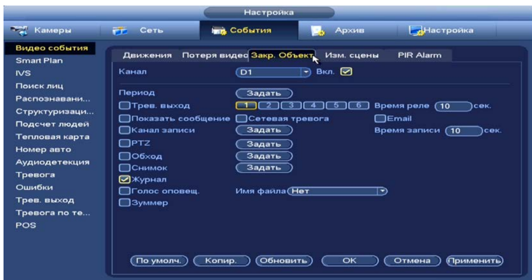
Рисунок 14.6 – Настройка события
