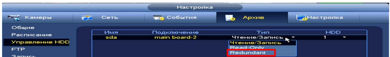
Рисунок 15.2 – Управление HDD
