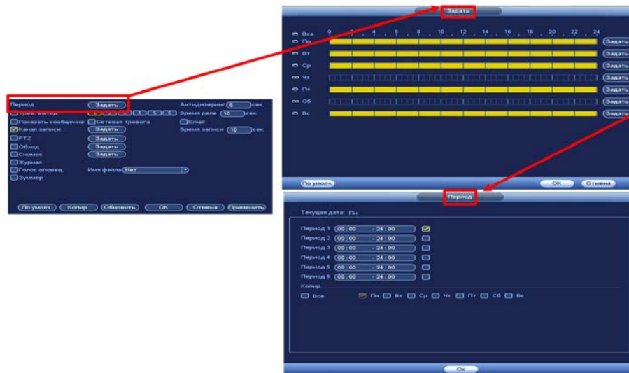
Рисунок 20.2 – Расписание
