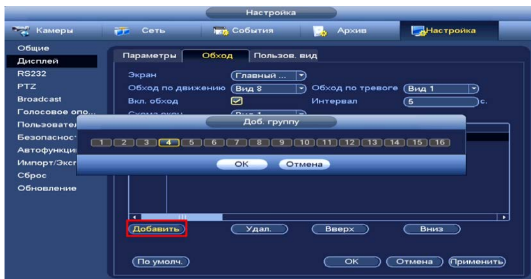
Рисунок 8.7 – Добавление группы
