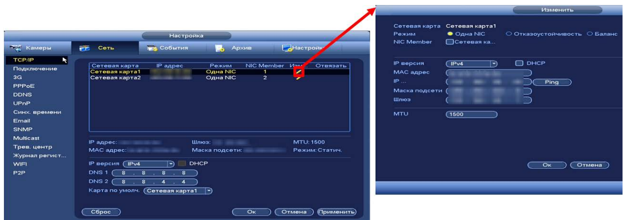
Рисунок 10.1 – Интерфейс настройки «ТСР/IP»
