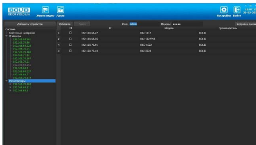
Рисунок 25.4 – Таблица результатов
