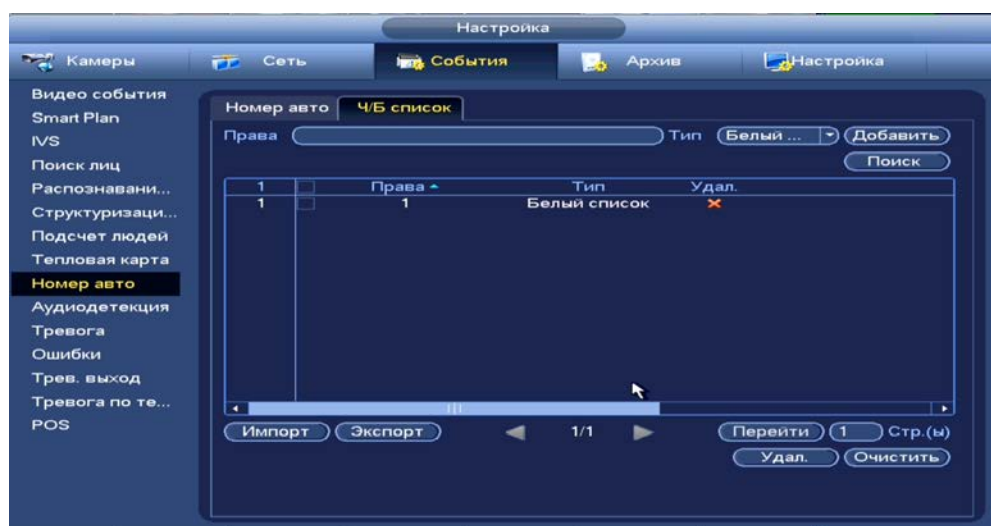
Рисунок 18.27 – Ч/Б список
