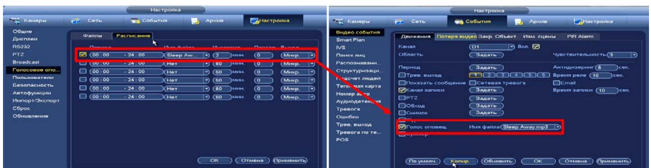
Рисунок 9.2 – Расписание
