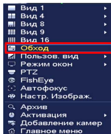
Рисунок 6.2 – Контекстное меню
