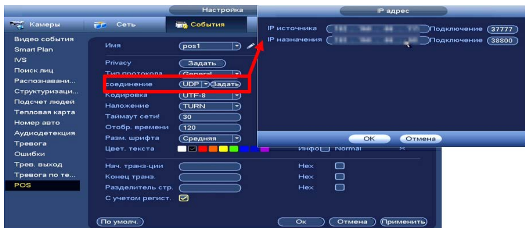
Рисунок 14.18 – POS функция
