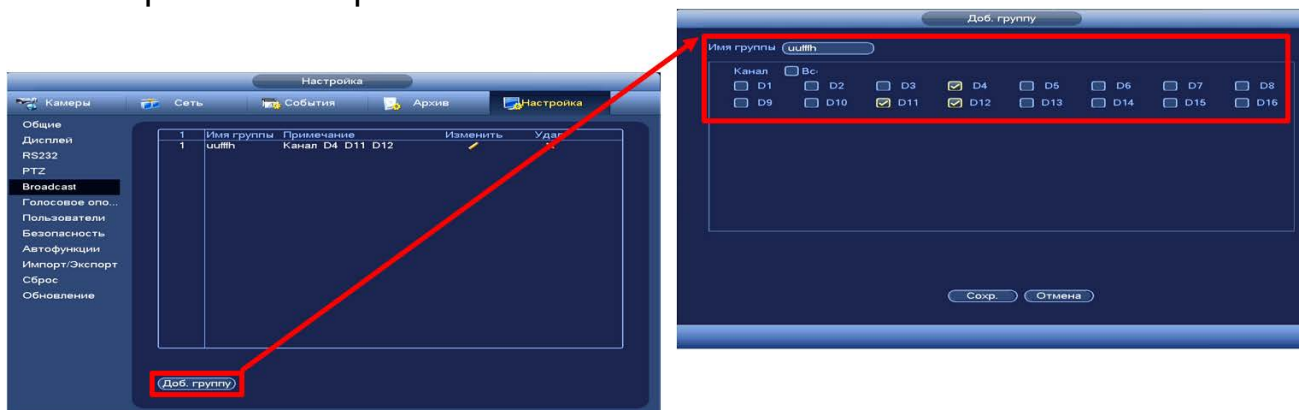
Рисунок 9.3 – Создание группы
