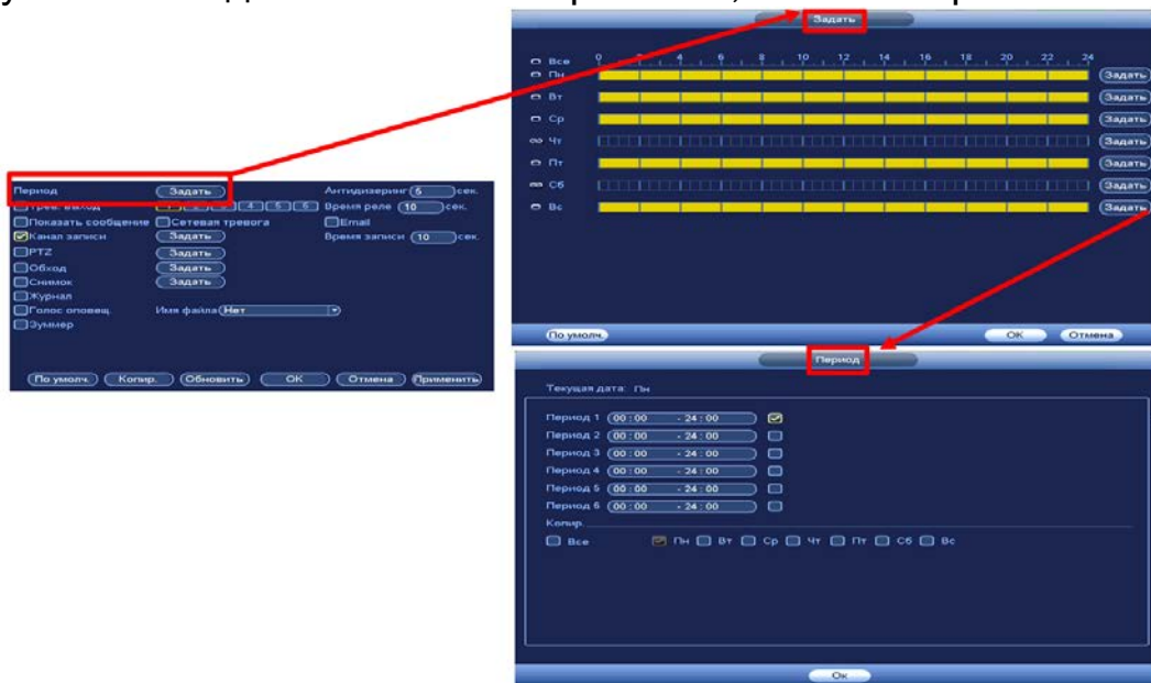
Рисунок 14.3 – Расписание
