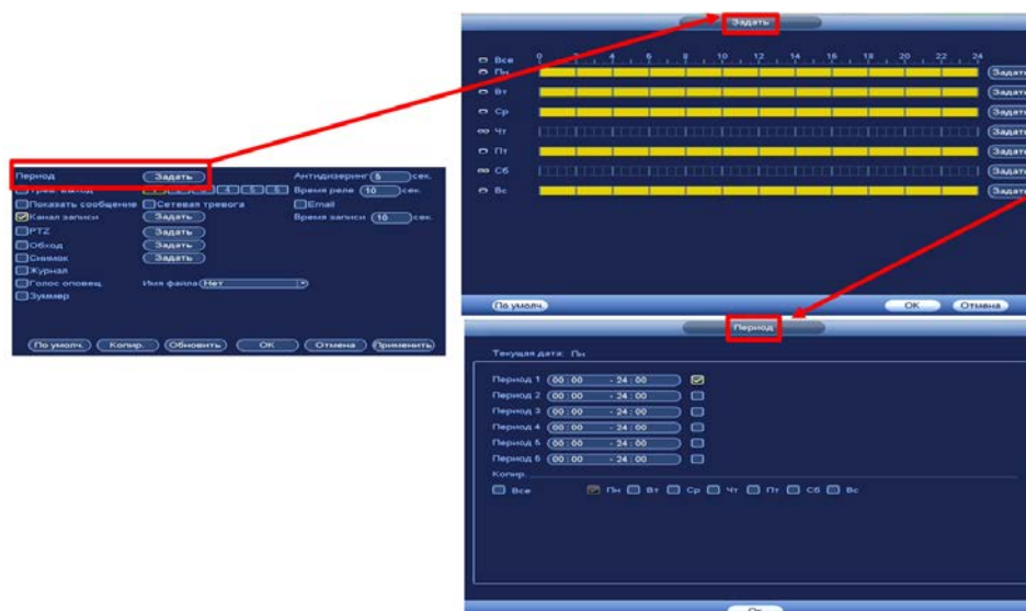
Рисунок 14.5 – Расписание
