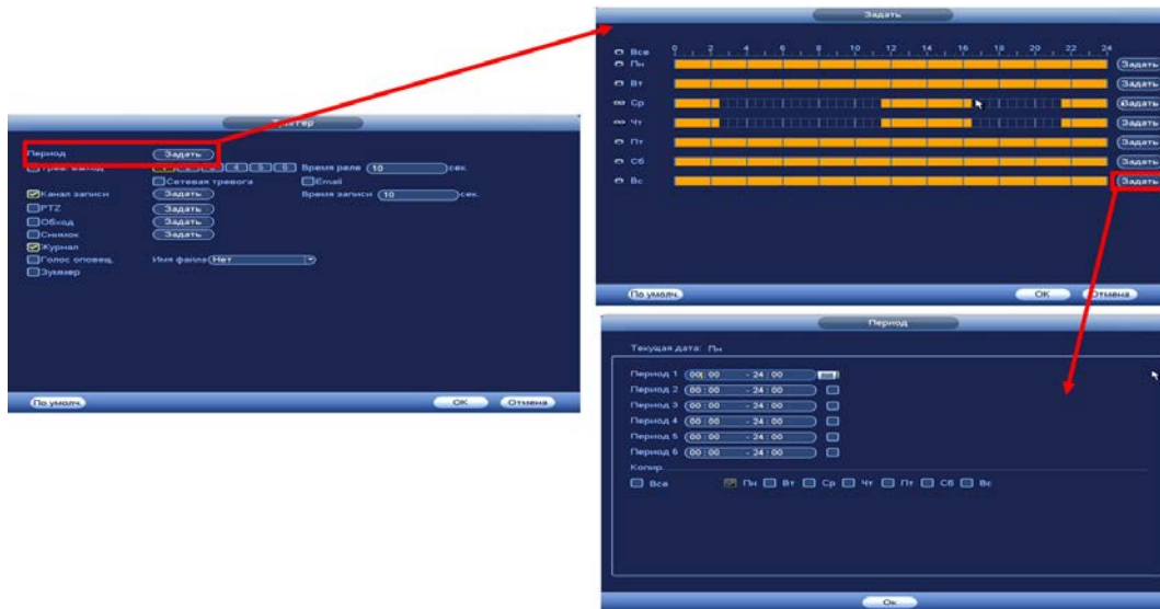
Рисунок 18.13 – Расписание
