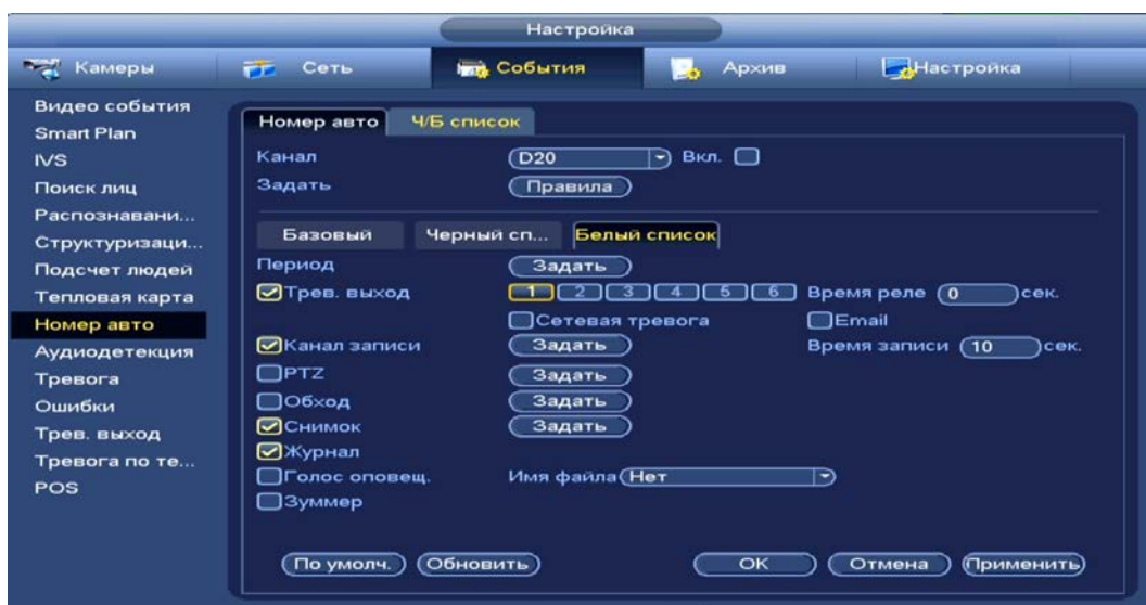
Рисунок 18.25 – Номер авто
