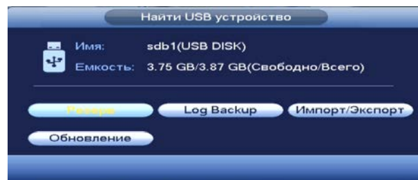
Рисунок 21.7 – Всплывающее окно при подключении USB-устройства
