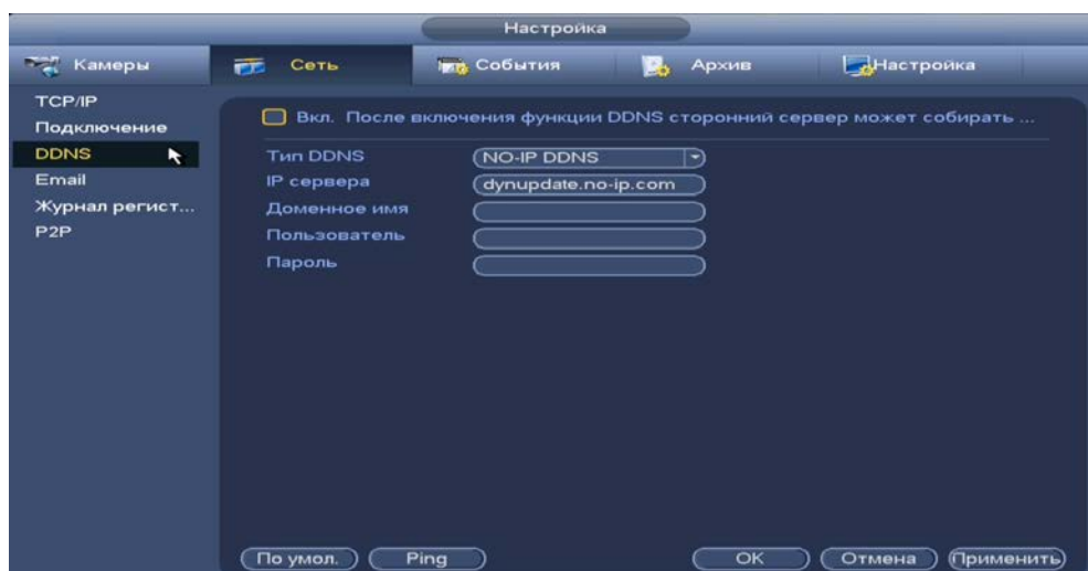
Рисунок 9.3 – Интерфейс настройки «DDNS»
