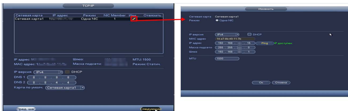
Рисунок 5.4 – Интерфейс настройки «TCP/IP»
