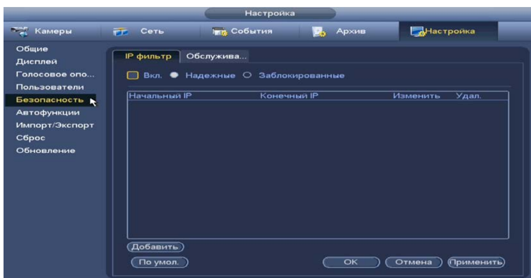
Рисунок 16.9 – Доступ
