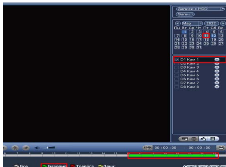
Рисунок 15.4 – Просмотр архива
