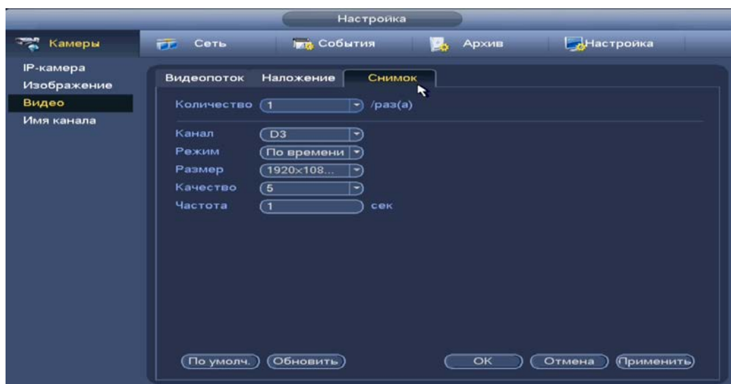
Рисунок 12.4 – Настройка снимка
