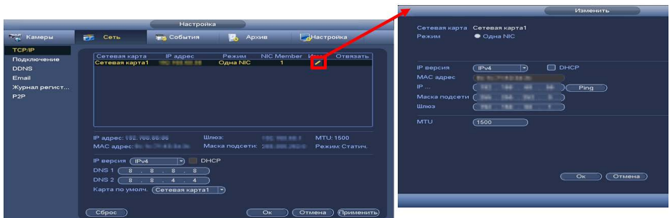
Рисунок 9.1 – Интерфейс настройки «ТСР/IP»
