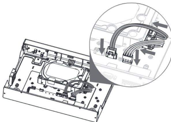
Рисунок 3.6 – Установка жесткого диска
