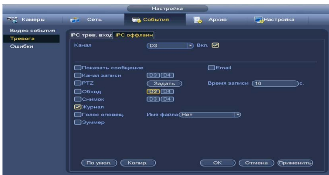
Рисунок 17.3 – Интерфейс настройки
