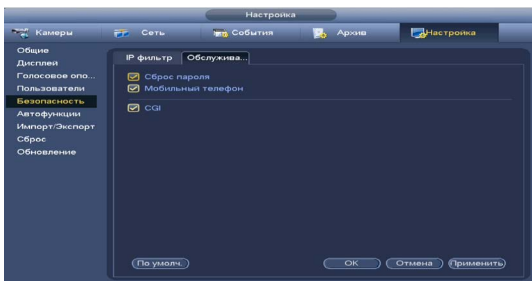
Рисунок 16.13 – Системное обслуживание
