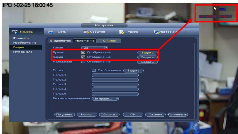
Рисунок 12.5 – Наложенные параметры
