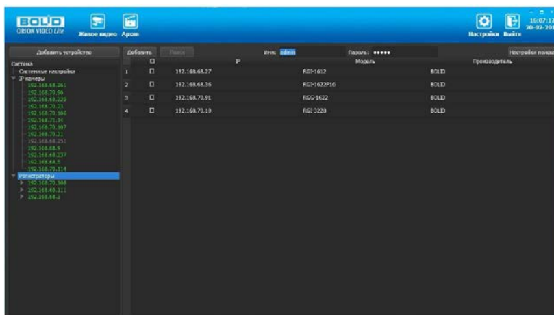
Рисунок 22.4 – Таблица результатов
