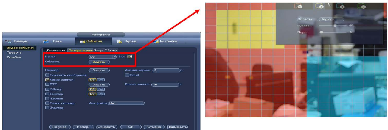
Рисунок 13.1 – Настройка области
