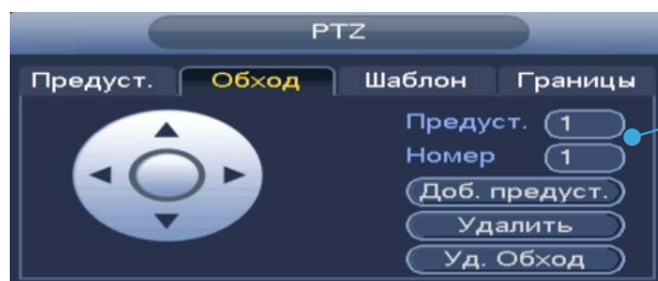
Рисунок 6.9 – Интерфейс «Обход»
